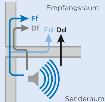
Schallübertragungswege vertikal
