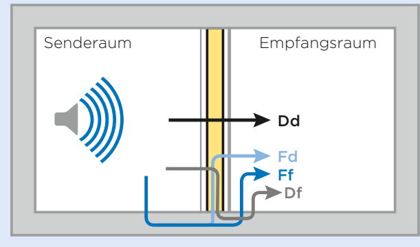
Schallübertragungswege horizontal
