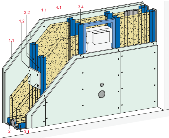
Systemskizze
