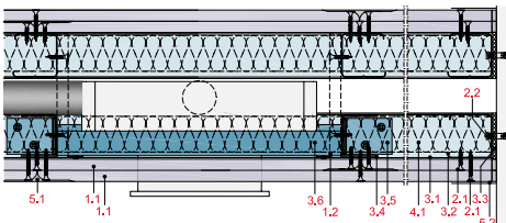
Längsschnitt
