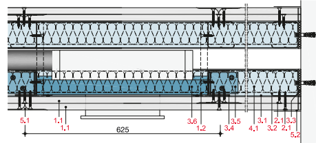
Längsschnitt
