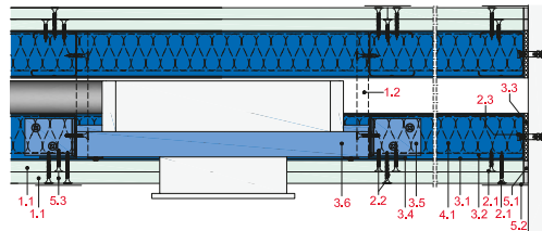
Längsschnitt
