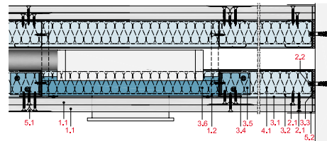
Längsschnitt
