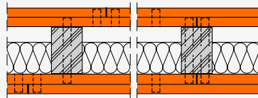
fermacell Montagewand mit Hohlraumdämmung als Einfachständerwand, zweilagig bekleidet
