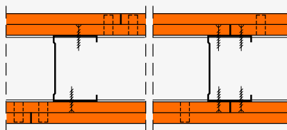
fermacell Montagewand ohne Hohlraumdämmung als Einfachständerwand, doppellagig bekleidet. Äußere Plattenlagen in 1./untere Plattenlagen geklammert
