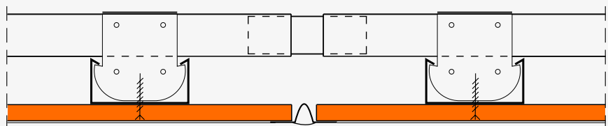
fermacell Decken-/Dachkonstruktion ohne Brandschutzanforderung. Bewegungsfuge mit Zusatzprofil.
