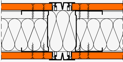
fermacell Montagewand, einlagig bekleidet, ohne Brandschutzanforderung. Bewegungsfuge mit Zusatzprofil
