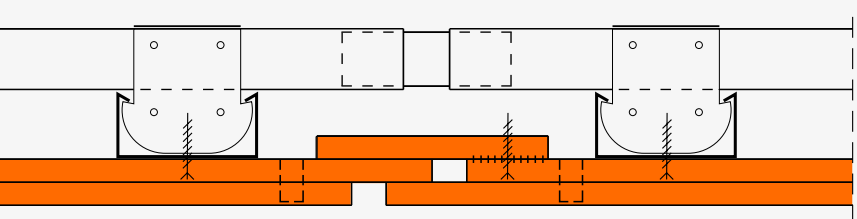
fermacell Decken-/Dachkonstruktion mit Brandschutzanforderung. Bewegungsfuge bei ein- bzw. zweilagiger Bekleidung. Plattenstreifen einseitig geklebt und verschraubt.
