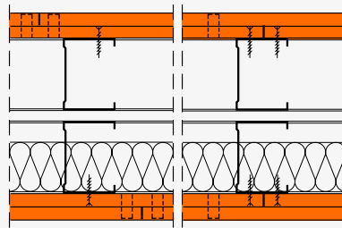
fermacell Montagewand als Doppelständerwand, zweilagig bekleidet. 2./äußere Plattenlage in 1./untere Plattenlage geklammert
