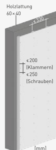
Wandkonstruktion mit Holzlattung, direkt befestigt
