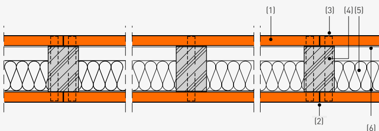
fermacell Montagewand mit Stahl-/Holzunterkonstruktion
