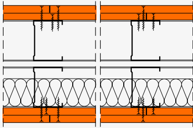
fermacell Montagewand als Doppelständerwand, zweilagig bekleidet. Beide Plattenlagen in Ständerprofile verschraubt
