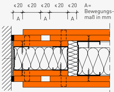
fermacell Montagewand, zweilagig bekleidet, F 90-A. Gleitender Wand- und/oder Fassadenanschluss mit zwei CW-Profilen und Plattenstreifen
