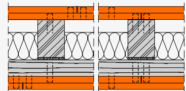
fermacell Montagewand mit Hohlraumdämmung als Einfachständerwand mit Querhölzern, doppelartig bekleidet
