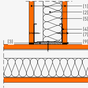
Wandverbindungen in T-Form bei ein- und zweilagiger Bekleidung, CW-Profil in fermacell Platte verschraubt
