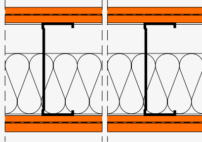
fermacell Brandwand tragend 4 ST 33
