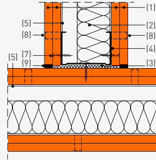
Wandverbindungen in T-Form bei ein- und zweilagiger Bekleidung, CW-Profil in fermacell Platte verschraubt
