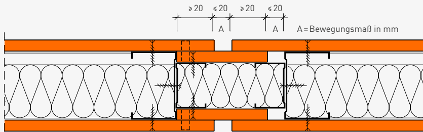
fermacell Montagewand, einlagig bekleidet, F 30-A/F 60-A. Bewegungsfuge mit Plattenstreifen
