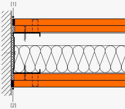
Wand- und Deckenanschlüsse mit zweilagiger fermacell Bekleidung
