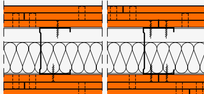
fermacell Montagewand mit Hohlraumdämmung als Einfachständerwand, dreilagig bekleidet. 2.+3. Plattenlage in 1. untere Plattenlage geklammert
