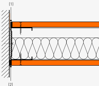
Wand- und Deckenanschlüsse mit einlagiger fermacell Bekleidung
