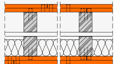
fermacell Montagewand mit Hohlraumdämmung als Doppelständerwand, doppelartig bekleidet
