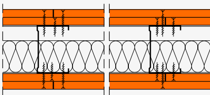
fermacell Montagewand als Einfachständerwand, doppellagig bekleidet. Beide Plattenlagen in Ständerprofile verschraubt
