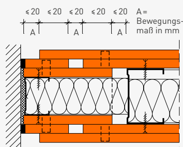
fermacell Montagewand, zweilagig bekleidet, F 90-A. Gleitender Wand- und/oder Fassadenanschluss mit einem CW-Profil und Plattenstreifen
