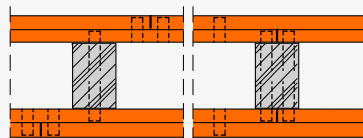
fermacell Montagewand ohne Hohlraumdämmung als Einfachständerwand, zweilagig bekleidet
