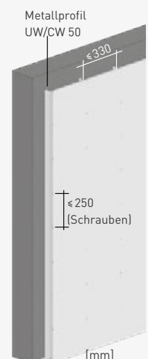
Wandkonstruktion mit Metallprofilen als Vorsatzschale
