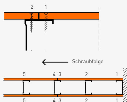
Anordnung der Plattenstöße bei einlagiger fermacell Bekleidung
