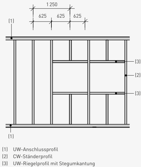
Ausbildung von Glasfeldöffnungen in der fermacell Montagewand (Maße in mm)
