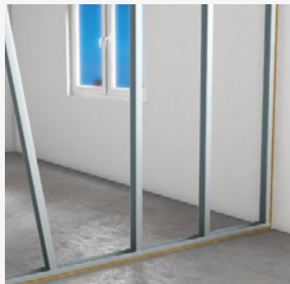
Montage der CW-Ständerprofile
