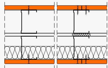
fermacell Montagewand als Doppelständerwand, einlagig bekleidet. CW-Profile getrennt angeordnet (links) bzw. durch selbstklebende Dämmstreifen (rechts) verbunden
