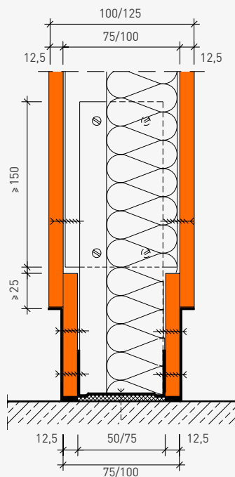
Zurückgesetzter Sockel bei einlagiger Bekleidung mit fermacell (Maße in mm)
