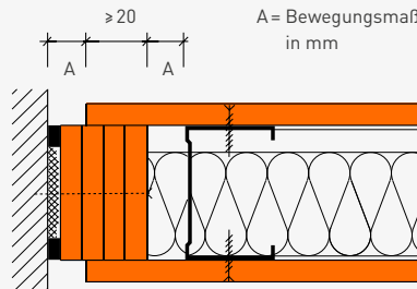
fermacell Montagewand, einlagig bekleidet, F 30-A/F 60-A. Gleitender Wand- und/oder Fassadenanschluss mit Streifenbündel
