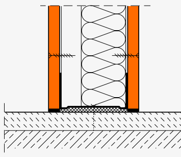
Trennwand auf Verbundestrich [R_{L,w,R}] = 38 bzw. 44 \text{ dB}^*
