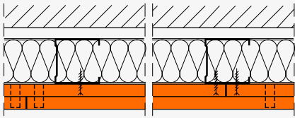
fermacell Vorsatzschale, zweilagig bekleidet
