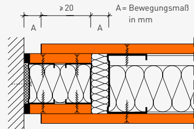
fermacell Montagewand, einlagig bekleidet, F 30-A/F 60-A. Gleitender Wand- und/oder Fassadenanschluss mit zwei CW-Profilen und Plattenstreifen
