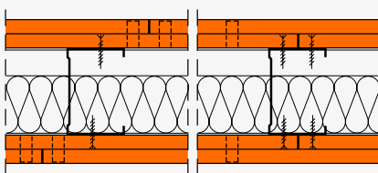
fermacell Montagewand als Einfachständerwand, doppellagig bekleidet. Äußere Plattenlagen in 1./untere Plattenlagen geklammert
