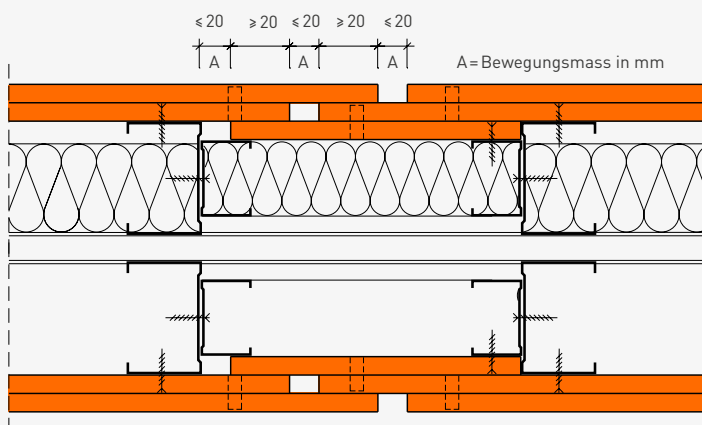
fermacell Montagewand als Doppelständerwand, zweilagig bekleidet, F 90-A. Bewegungsfuge mit Plattenstreifen
