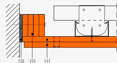
Anschluss mit Streifenbündel
