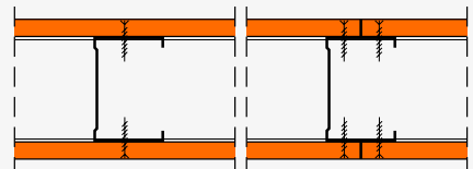
fermacell Montagewand ohne Hohlraumdämmung als Einfachständerwand, einlagig bekleidet
