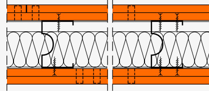
Hoch schalldämmende fermacell Montagewand, doppelartig bekleidet
