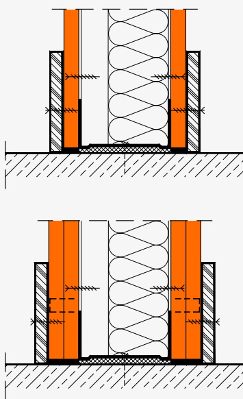
Aufgesetzter Sockel bei einlagiger/zweilagiger Bekleidung mit fermacell
