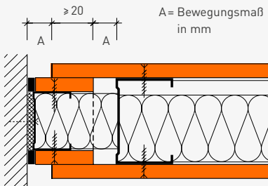
fermacell Montagewand, einlagig bekleidet, F 30-A/F 60-A. Gleitender Wand- und/oder Fassadenanschluss mit einem CW-Profil und Plattenstreifen
