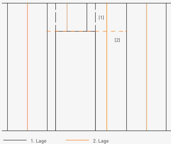
Bekleidungschema zweilagig bekleidete fermacell Montagewand
