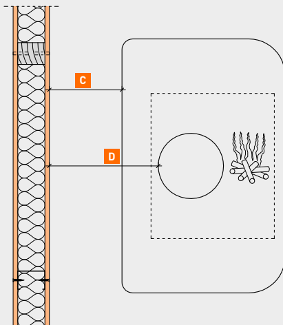
Abstände Öfen vor Holztafelbauwand
