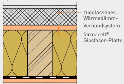
Wirksamer Wetterschutz WDVS
