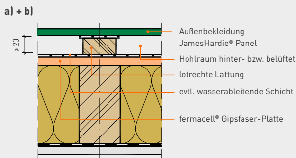
Dauerhaft wirksamer Wetterschutz a) hinter- bzw. b) belüftet
