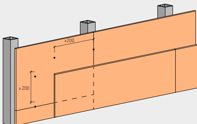
Versetzen der zweiten Lage bei mehrlagiger Beplankung
