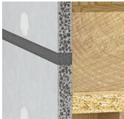
Bild 4: Verschließen der Fuge mit einem vorkomprierten Dichtungsband (Detail)
