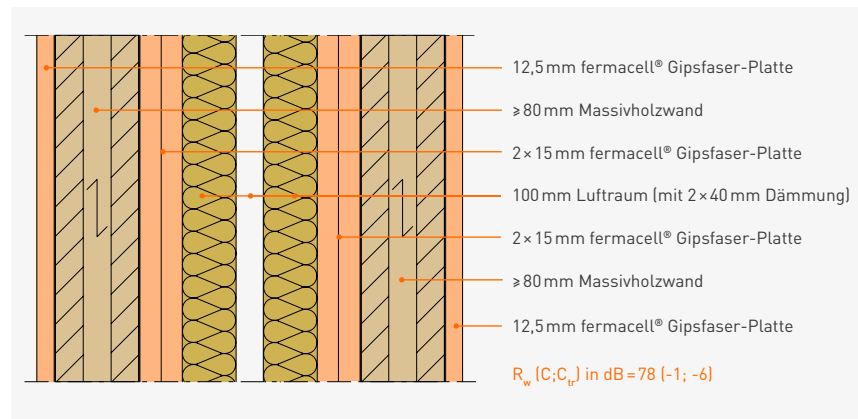
Gebäudeabschlusswand – tieffrequenter Einsatz (Beispiel)
