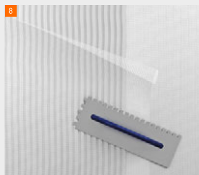
Überlappung des Armierungsgewebes mit ca. 100 mm
