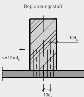
Bild 4: Erforderliche Randabstände für Klammern
