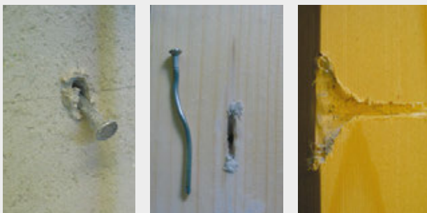
Plastische Verformung und Lochaufweitung nach der zyklisch-dynamischen Beanspruchung der Konstruktion. fermacell® Gipsfaser-Platten (links), Holzunterkonstruktion mit verformtem Verbindungsmittel (Mitte), Schnitt durch Holzunterkonstruktion (rechts)
