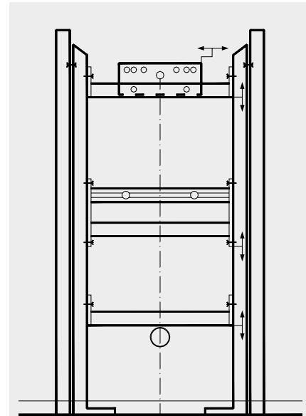
Tragständer für Waschbecken, Urinale oder Ausgüsse
