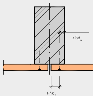
Bild 6: Abstände bei einer Mittelrippe/Nägel
