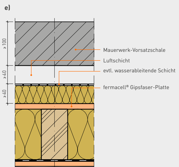
Dauerhaft wirksamer Wetterschutz Mauerwerk-Vorsatzschale
