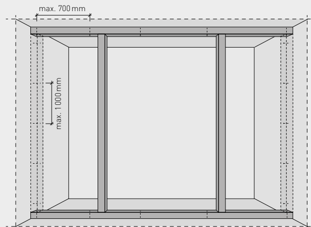
Befestigungsabstände
