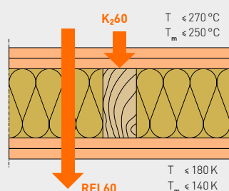
Beispiel Gebäudeklasse 4: Ausführung einer Holzständerwand (REI 60/K 2 60) gemäß den Anforderungen der Muster-Richtlinie (M-HFHHolzR)/hochfeuerhemmendes Bauteil
