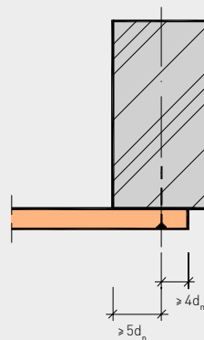
Bild 8: Abstände bei einer Randrippe/Nägel
