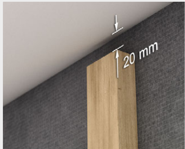
Mindestabstand zwischen Oberkante Traglattung und oberem Abschluss.
