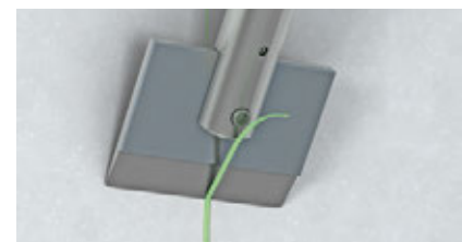
Entfernen des überschüssigen Klebers mit fermacell™ Klebstoffabstoßer
