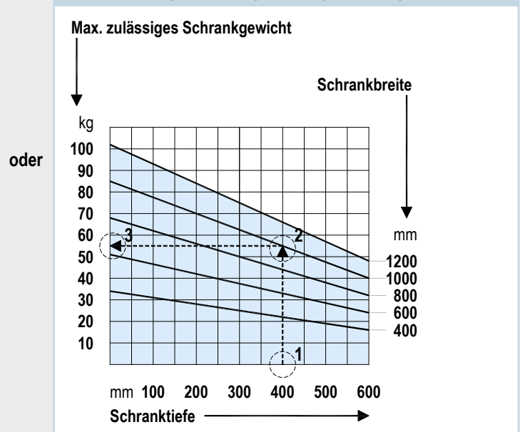
Maximal zulässiges Schrankgewicht (kg) nach Diagramm
