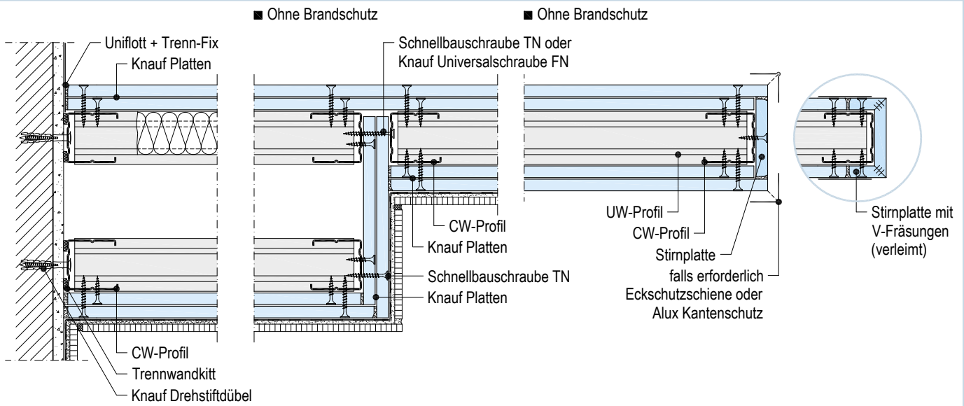
W116.de-A1 Anchl. an Massivw. W116.de-D1 Wandverjüngung
